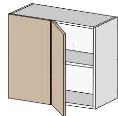
Upper Return Door*
